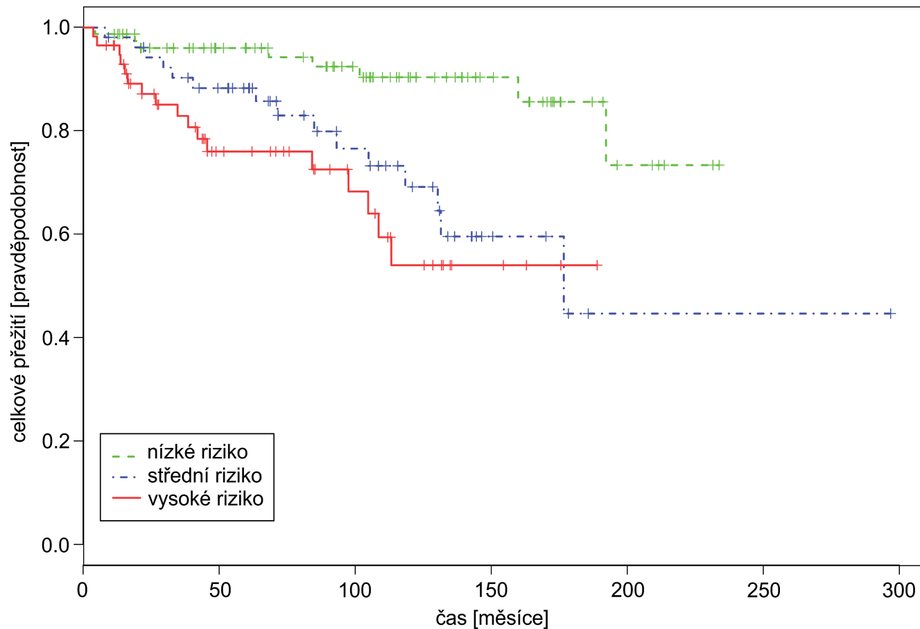
Obr. 4 Celkové přežití pacientů podle nového skóre vytvořeného součtem Hasfordova skóre (1–3 body) a Sokalova skóre (1–3 body). Populace byla rozdělena na tři kategorie: nízké riziko (Has+Sok \leq 3 ), střední riziko (Has+Sok = 4) a vysoké riziko (Has+Sok \geq 5 ). Konkordance C_{\text{HAS+SOK}} = 0,674 ; rozdíl mezi středně a nízkou rizikovou skupinou byl statisticky významný HR_{(\text{HAS+SOK}2)} = 3,41 , p = 0,006 , rozdíl mezi vysoko a nízkou rizikovou skupinou taktéž HR_{(\text{HAS+SOK}3)} = 5,00 , p < 0,001 .
