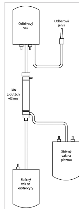
Obr. 2 Schéma „BCC“ s filtrem z dutých vláken.
