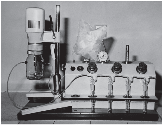
Obr. 3. Prístroj na izoláciu alveolárneho vzduchu UZBL 1.
