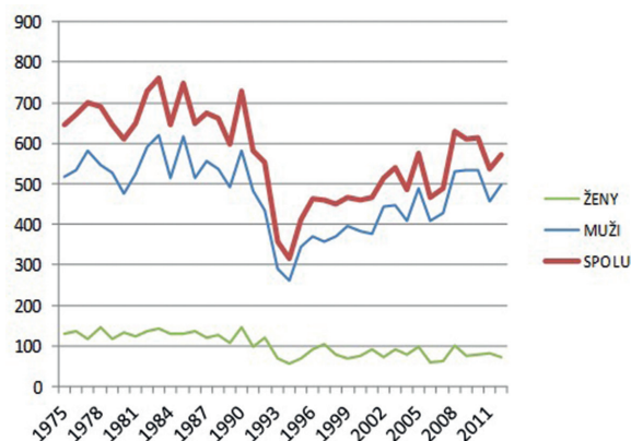
Obr. 2. Vývoj počtu samovrážd v SR (1975-2012).
