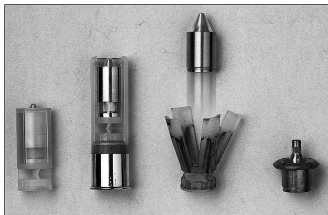
Obr. 3. Podkaliberní střela Brenneke SuperSabot (Brenneke®). Zleva doprava: střela v plastovém obalu, střela s pouzdrům v nábojnici, střela krátce po opuštění hlavně a deformace střely při zásahu cíle
