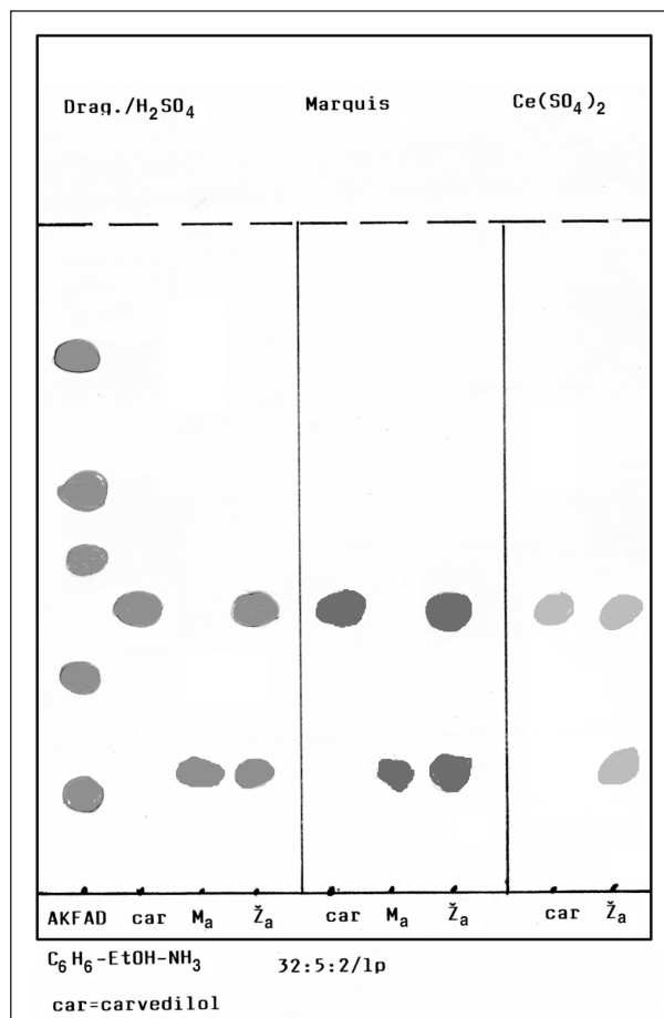
Obr. 12. Carvedilol
