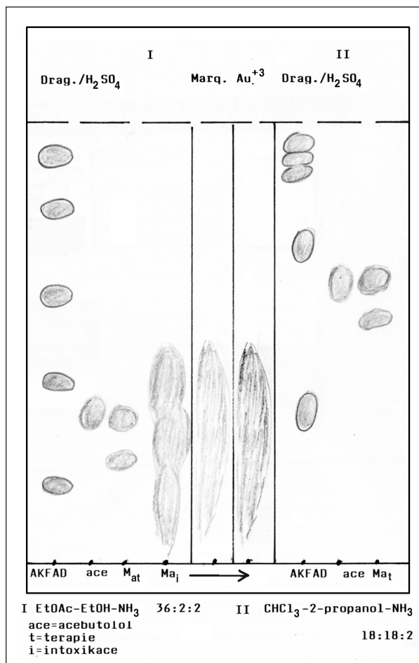
Obr. 10. Acebutolol
