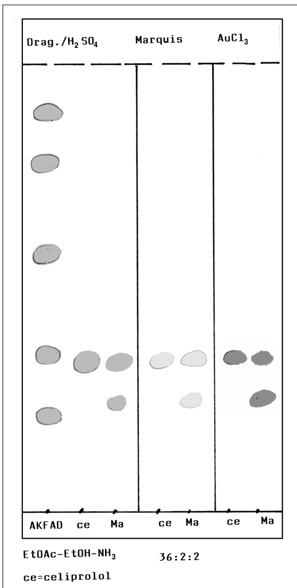
Obr. 11. Celiprolol
