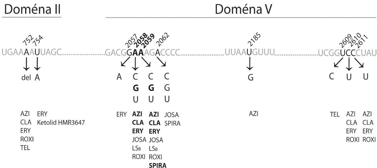
Obr. 2. Mutace vlásenky 35 domény II (mezi koordinátami 737-760) a centrální smyčky domény V (mezi koordinátami 2000-2624) molekuly 23S rRNA vedoucí k rezistenci k různým makrolidovým antibiotikům. Zobrazené mutace byly popsány u rodů Brachyspira , Campylobacter , Escherichia , Chlamydia , Lactobacillus , Mycobacterium , Mycoplasma , Neisseria , Propionibacterium , Pseudomonas , Staphylococcus , Streptococcus , Streptomyces , Treponema a Turicella . Zvýrazněné údaje se týkají TPA. Koordináty jsou uvedeny podle pozice ve 23S rRNA E. coli . AZI – azitromycin; CLA – klaritromycin; ERY – erytromycin; JOSA – josamycin; LSB – linkosamid a streptogramin B; ROXI – roxitromycin; SPIRA – spiramycin; TEL – telitromycin Fig. 2. Mutations in hairpin 35 of domain II (coordinates 737-760) and the central loop of domain V (coordinates 2000-2624) of the 23S rRNA molecule conferring resistance to different macrolides. Such mutations have been reported in the genera Brachyspira , Campylobacter , Escherichia , Chlamydia , Lactobacillus , Mycobacterium , Mycoplasma , Neisseria , Propionibacterium , Pseudomonas , Staphylococcus , Streptococcus , Streptomyces , Treponema , and Turicella . The data highlighted are related to Treponema pallidum subsp. pallidum (TPA). Coordinates are given in accordance with the positions in 23S rRNA of E. coli . AZI – azithromycin; CLA – clarithromycin; ERY – erythromycin; JOSA – josamycin; LSB – lincosamides and streptogramin B; ROXI – roxithromycin; SPIRA – spiramycin; TEL – telithromycin
