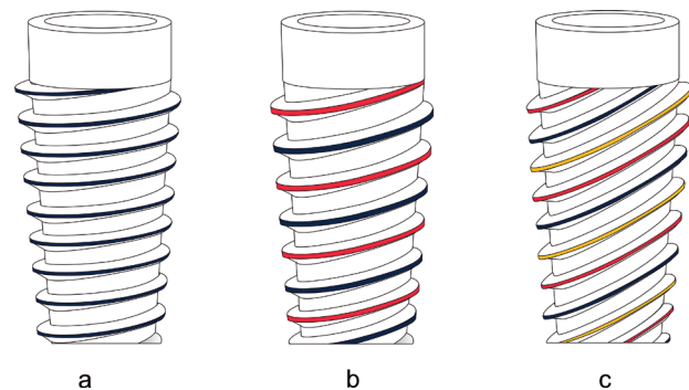
Obr. 3 Jednoduchý, dvojí a trojí závit; a) jednoduchý závit b) dvojí závit c) trojí závit
