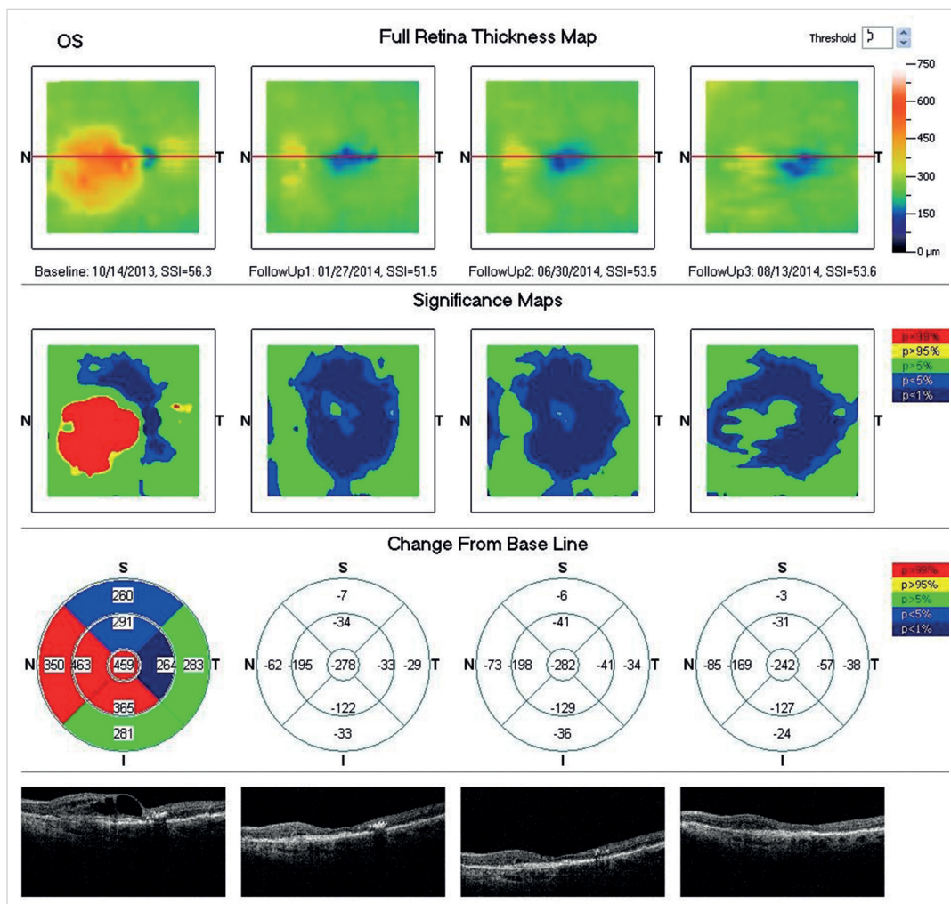
Obr. 10 OCT snímok (porovnávací – po 10 mesiacoch liečby afliberceptom). Regresia edému neuroretiny aj hrúbky sietnice – CHS: -242 μm
