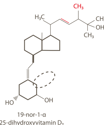
Parikalcitol
