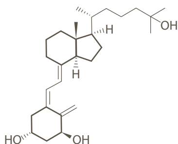
Kalcitriol
