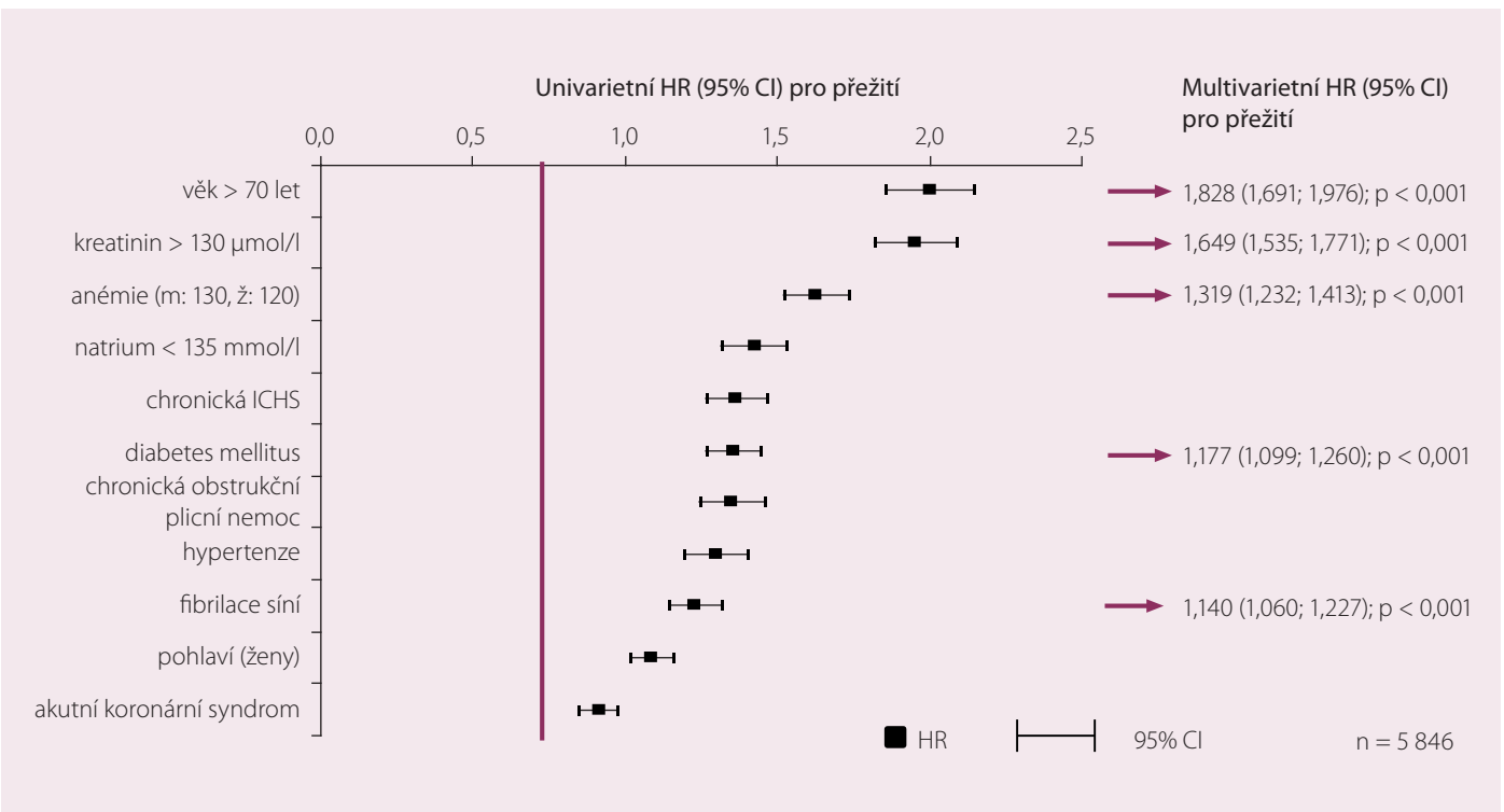
Obr. 4. Význam komorbidit pro mortalitu.
