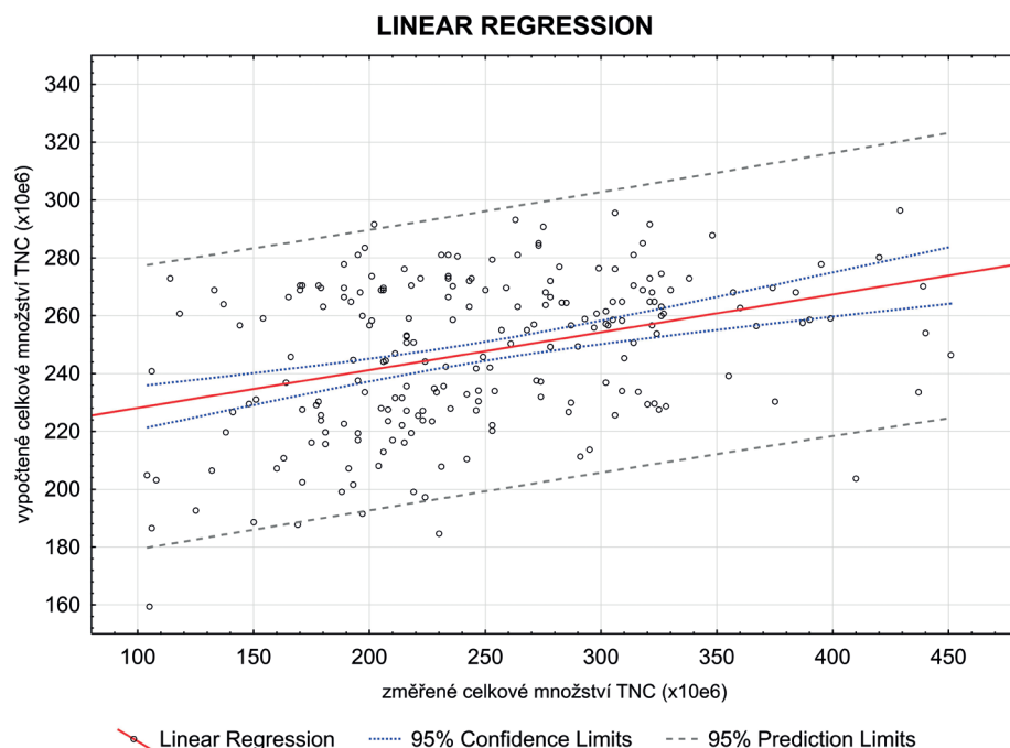
Graf 2. Porovnání vypočtených a skutečných výtěžků (TNC x 10 8 ), lineární regrese
