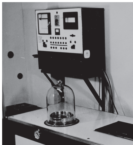
Obr. 2. Zariadenie na deštrukciu tkaniva a homogenizáciu alveolárneho vzduchu.
