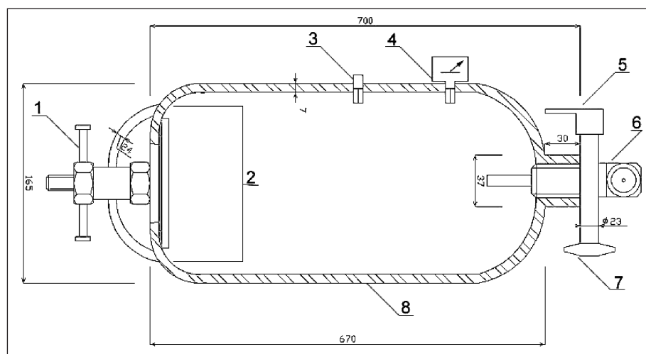
Obr. 1. Schéma konštrukcie experimentálnej pretlakovej komory 1 – vonkajšia časť uzáveru s kľúčovou matkou, 2 – vnútorná časť uzáveru fľaše, 3 – poistný pretlakový ventil, 4 – tlakomer, 5 – telo ventilu fľaše, 6 – INT/DIN pripojenie na ventil fľaše, 7 – regulátor napúšťania, 8 – telo komory
