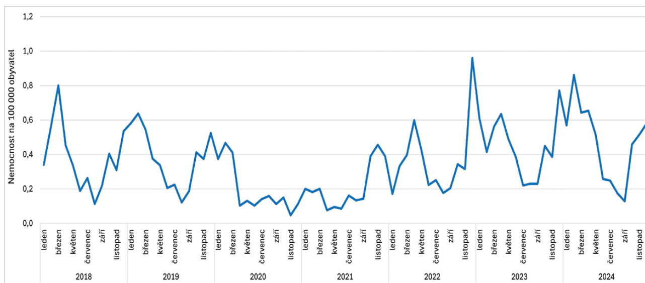
Obr. 2. Měsíční nemocnost IPO, 2018–2024, Česká republika, surveillance data
