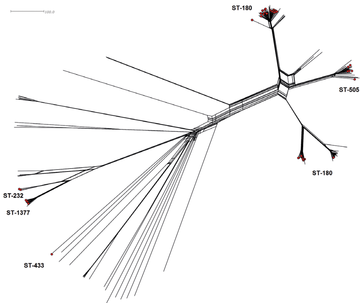
Obr. 7. Genetická diverzita českých (63 izolátů) a světových (176 izolátů) izolátů S. pneumoniae sérotypu 3 dostupných v PubMLST databázi za období 2018–2024 Figure 7. Genetic diversity of Czech (63 isolates) and global (176 isolates) S. pneumoniae serotype 3 isolates available in the PubMLST database for the period 2018–2024
