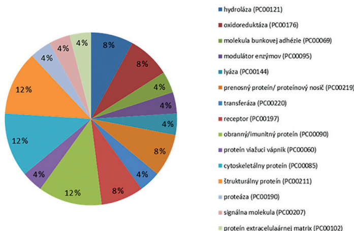
Graf 1 GO klasifikácia identifikovaných proteínov do proteínových tried Graph 1 GO classification of identified proteins into protein classes
