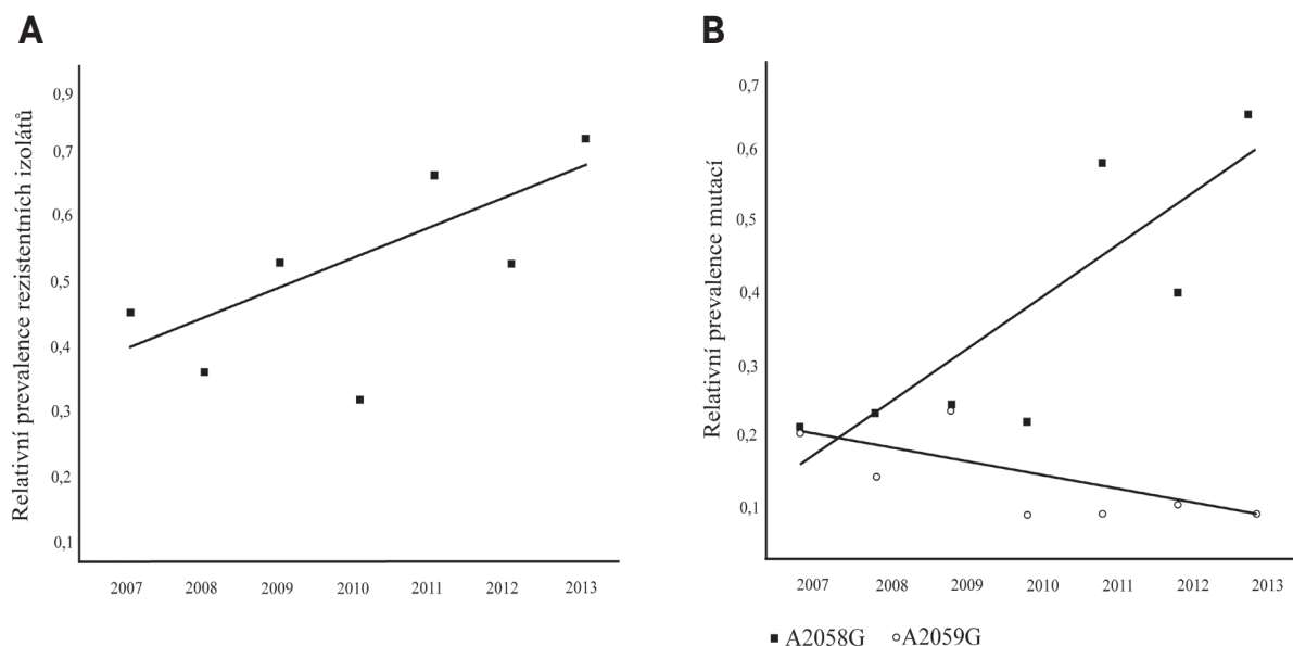
Obr. 3. Prevalence rezistentních izolátů a prevalence mutace A2058G a A2059G ve 23S rRNA genech TPA kmenů v ČR v letech 2007–2013. Spojnice trendu byla vytvořena pomocí programu MS Excel 2003.
