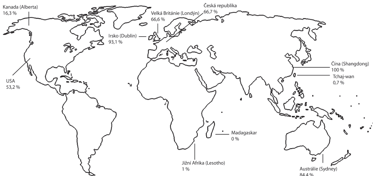
Obr. 4. Distribuce prevalence rezistentních kmenů TPA ve světě
