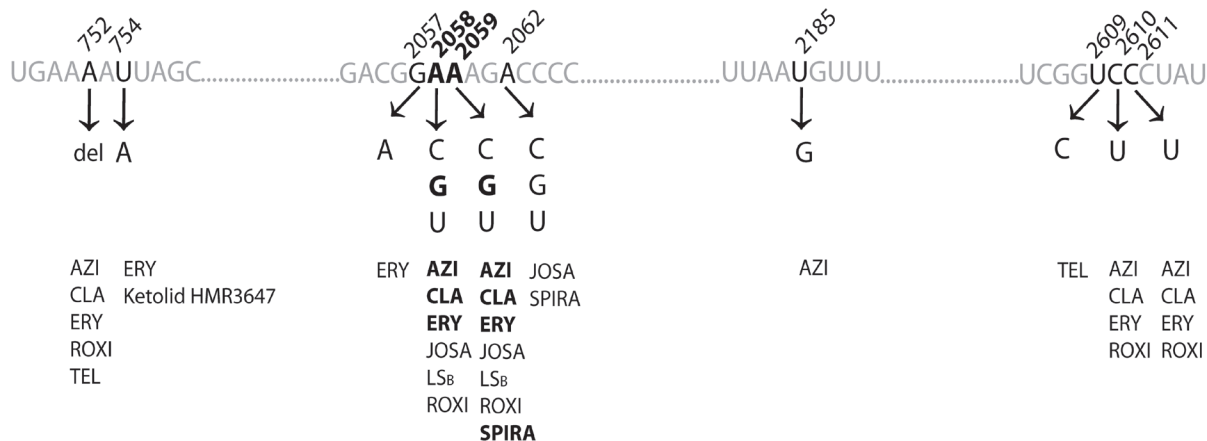
Obr. 2. Mutace vlásenky 35 domény II (mezi koordinátami 737-760) a centrální smyčky domény V (mezi koordinátami 2000-2624) molekuly 23S rRNA vedoucí k rezistenci k různým makrolidovým antibiotikům. Zobrazené mutace byly popsány u rodů Brachyspira , Campylobacter , Escherichia , Chlamydia , Lactobacillus , Mycobacterium , Mycoplasma , Neisseria , Propionibacterium , Pseudomonas , Staphylococcus , Streptococcus , Streptomyces , Treponema a Turicella . Zvýrazněné údaje se týkají TPA. Koordináty jsou uvedeny podle pozice ve 23S rRNA E. coli . AZI – azitromycin; CLA – klaritromycin; ERY – erytromycin; JOSA – josamycin; LSB – linkosamidy a streptogramin B; ROXI – roxitromycin; SPIRA – spiramycin; TEL – telitromycin.
